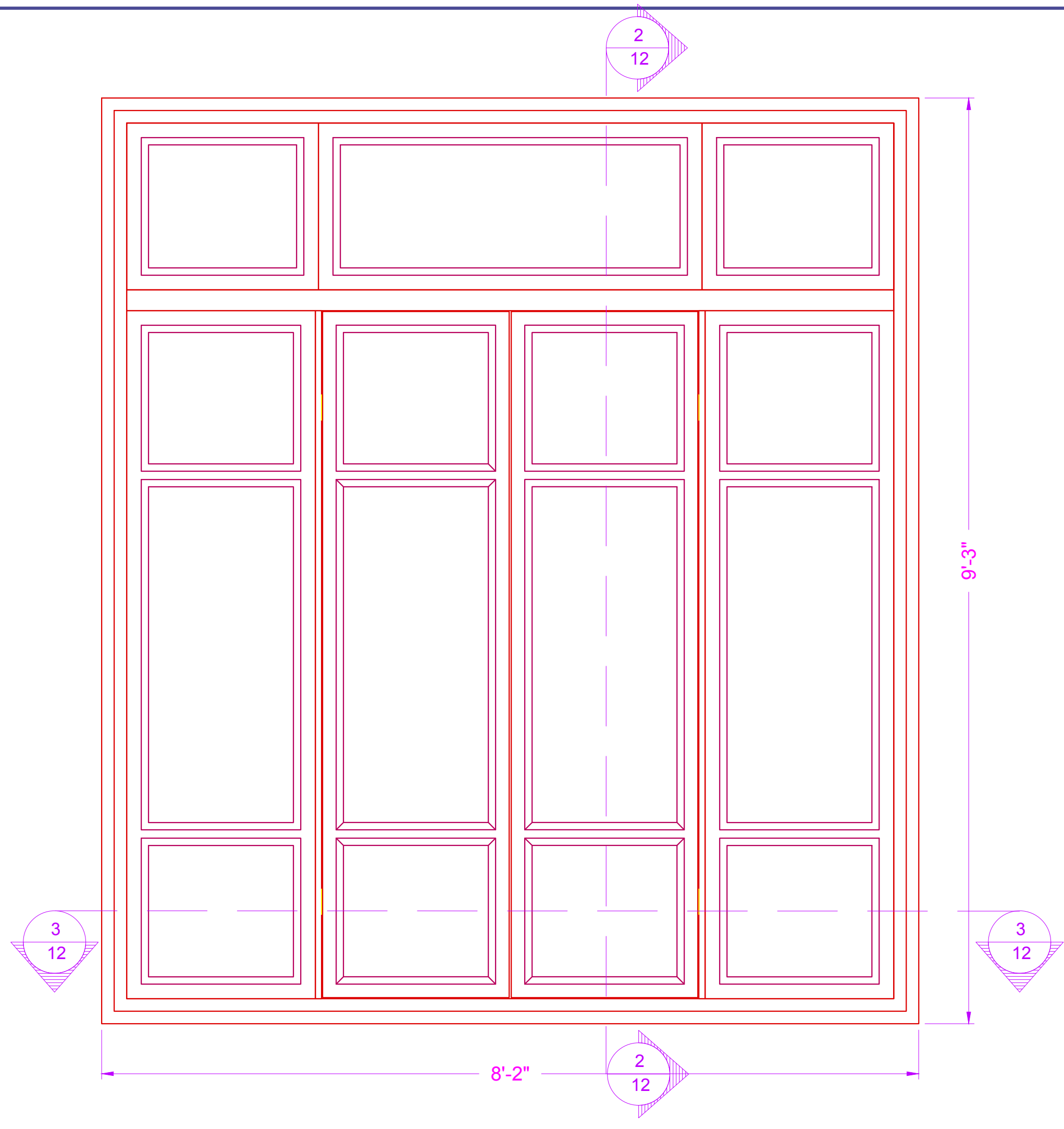
6 WINDOW - ASSEMBLED SCALE: 1"=1'-0"
