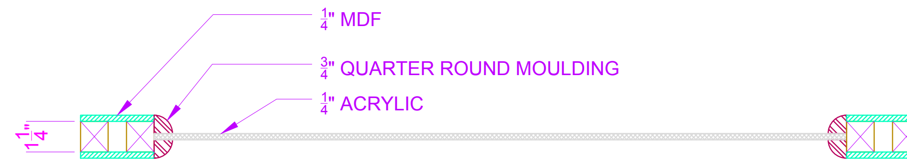
6 DOOR WALL - TRANSOM - SECTION VIEW SCALE: 3"=1'-0" QTY: (2)
