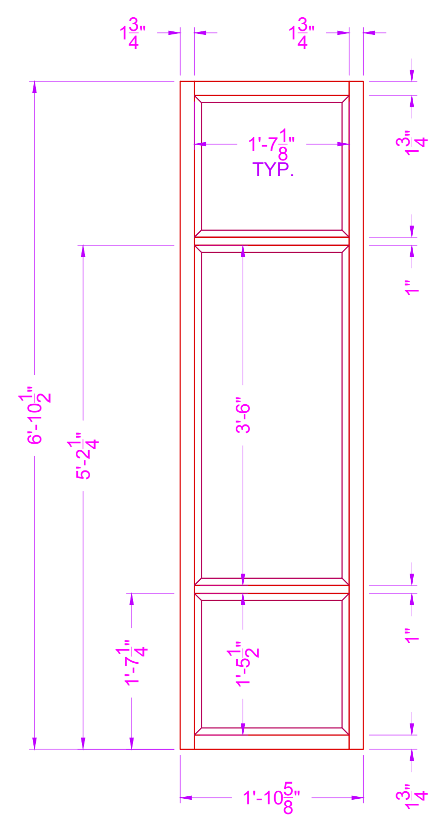
5 BOTTOM OUTER WINDOWS SCALE: 1/2"=1'-0" QTY: (2)
