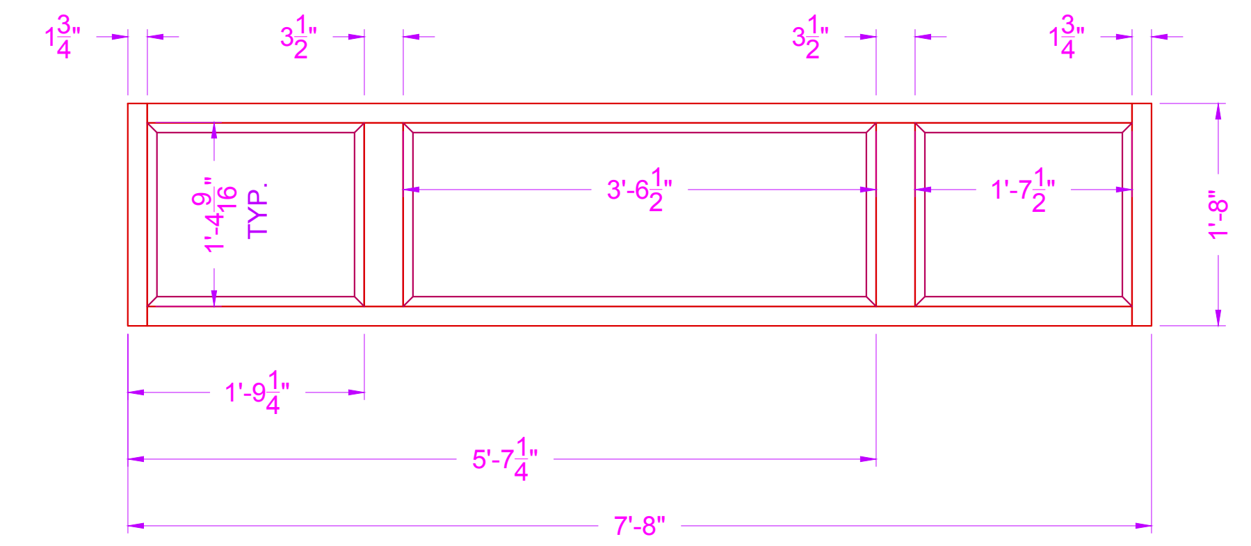
4 UPPER WINDOW SCALE: 1/2"=1'-0" QTY: (1)
